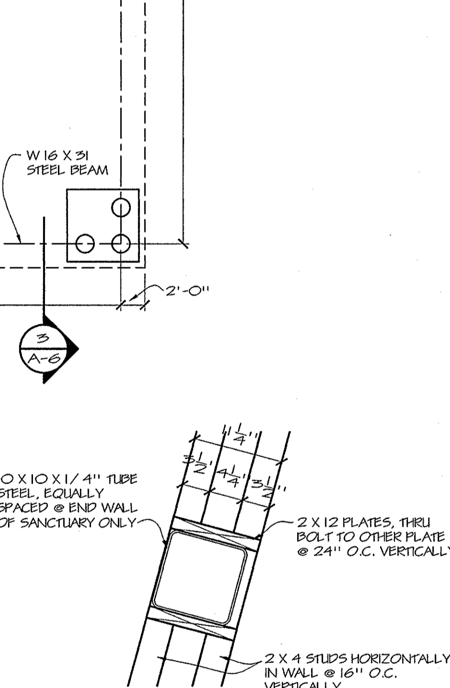
DETAIL 1 SCALE: 1/8" = 1'-0" FLOOR PLAN SCALE: 1/8" = 1'-0"
